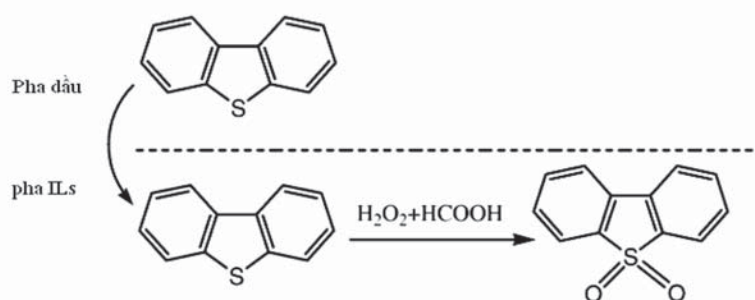
Hình 3. Quá trình oxy hóa loại dipenzothiophen sử dụng chất lỏng ion [BMIM][HSO 4 ] như là xúc tác chuyển pha [20]
